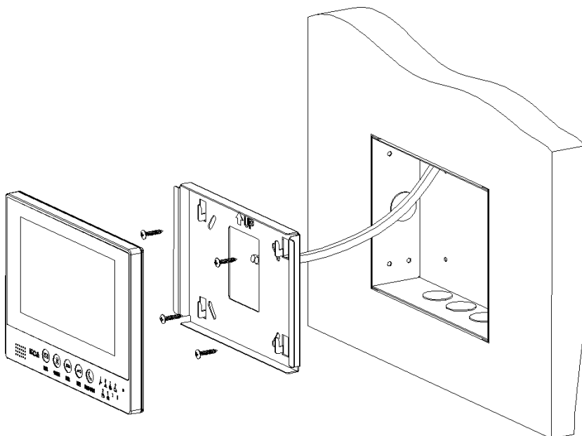
埋入式施工圖
