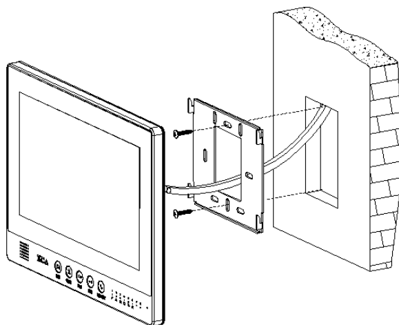
壁掛式施工圖
