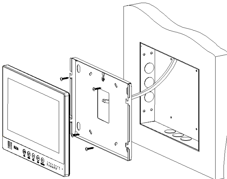
埋入式施工圖
