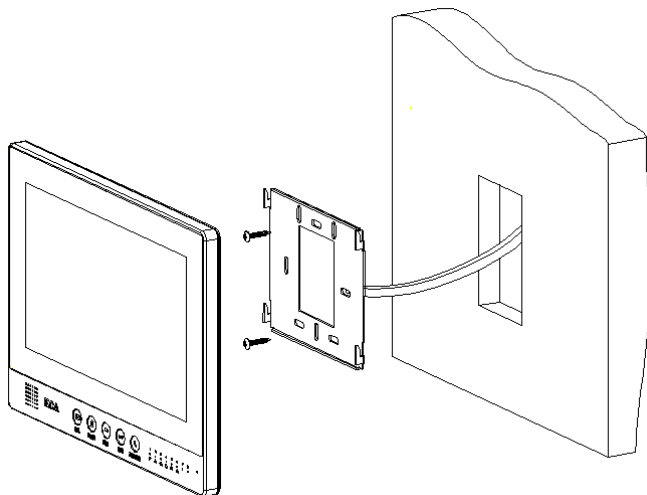
壁掛式施工圖
