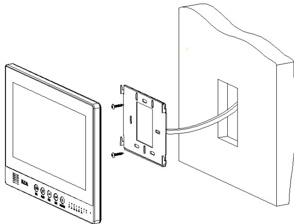
壁掛式施工示意圖
